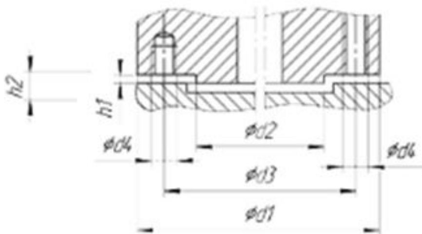
Присоединительные размеры пневмопривода DN150
