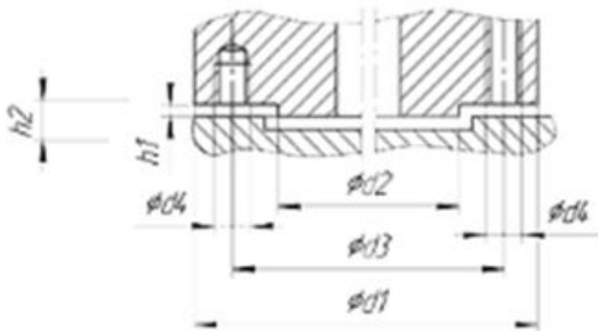
Присоединительные размеры пневмогидропривода DN200
