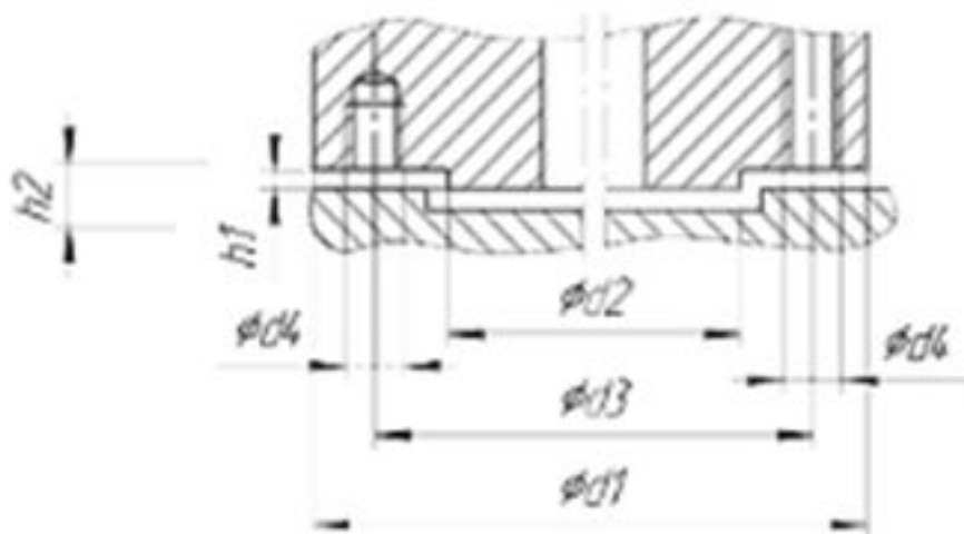
Присоединительные размеры пневмогидропривода DN300-400
