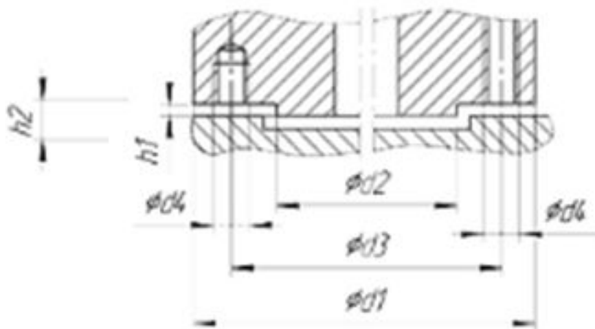
Присоединительные размеры пневмогидропривода DN300
