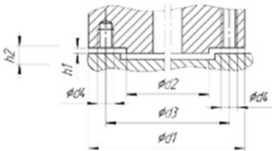
Присоединительные размеры пневмопривода DN50
