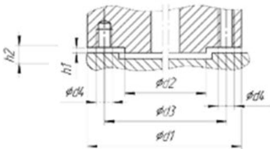
Присоединительные размеры пневмопривода DN80-100
